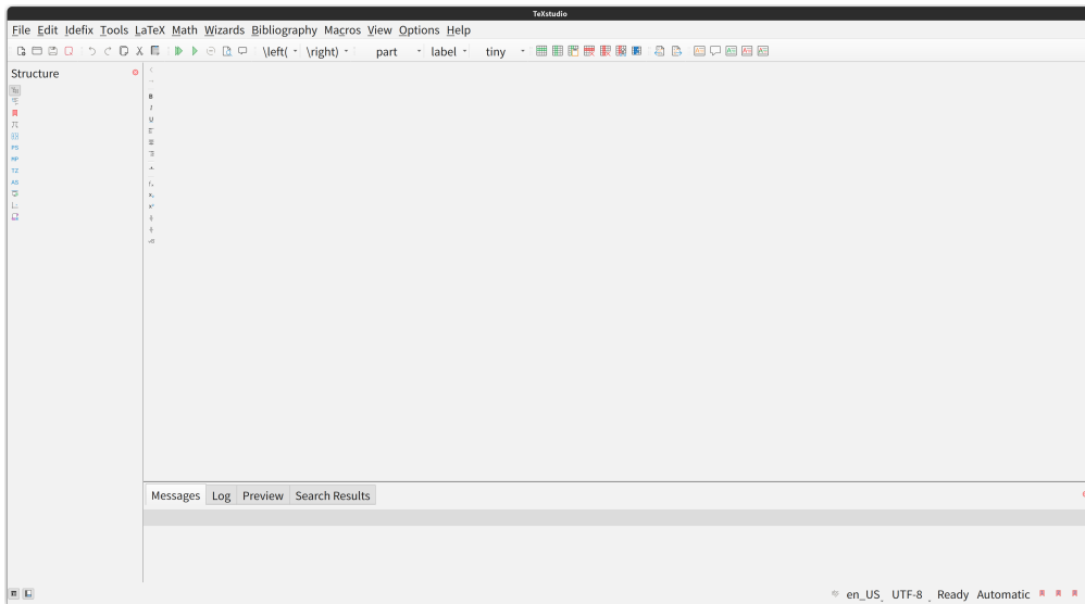
图 1.2 TeXstudio 界面
